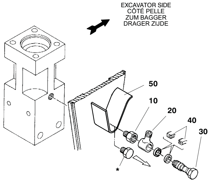
Gusset position Position du gousset Montagemaße für Schutzblech Stand van verbindingsplaat
